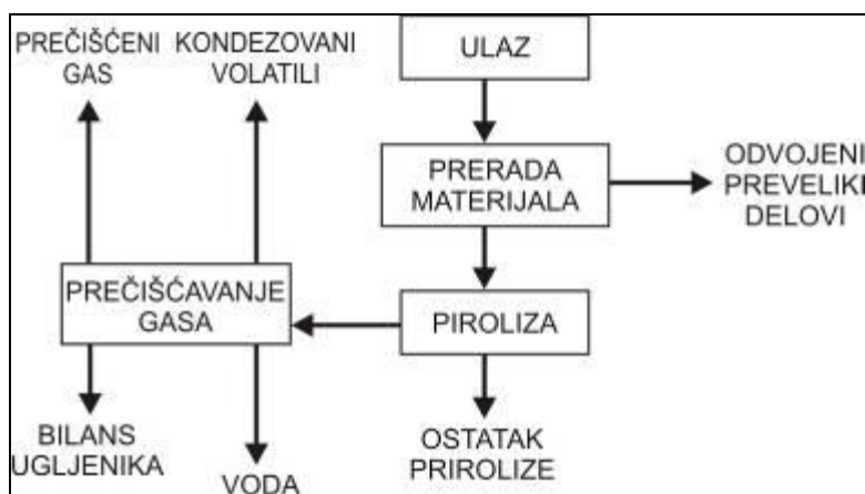
Slika 4.23. Šematski prikaz procesa pirolize
