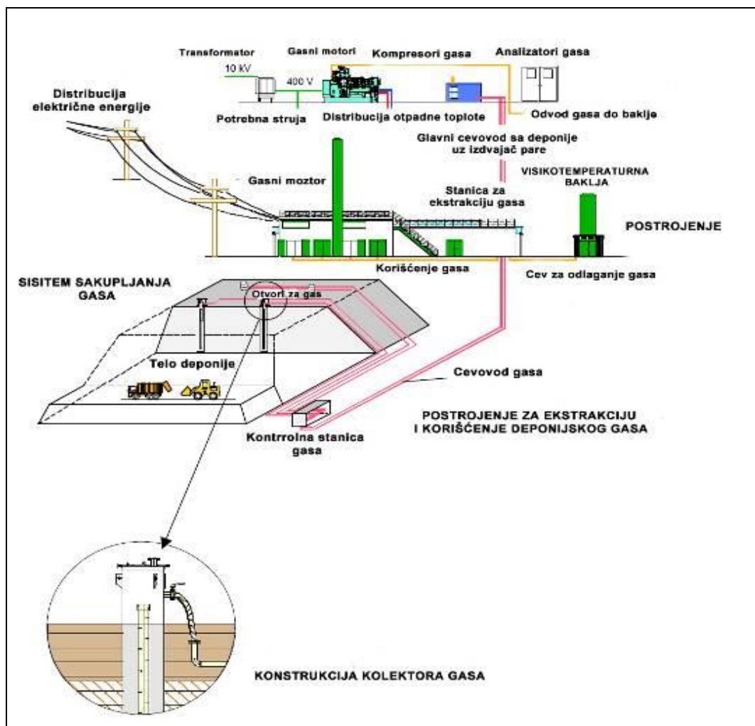
Slika 5.12. Šema toka deponijskog gasa kroz postrojenje
